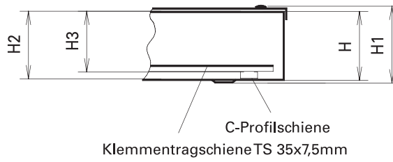
Abb. Gehäuse im Schnitt
