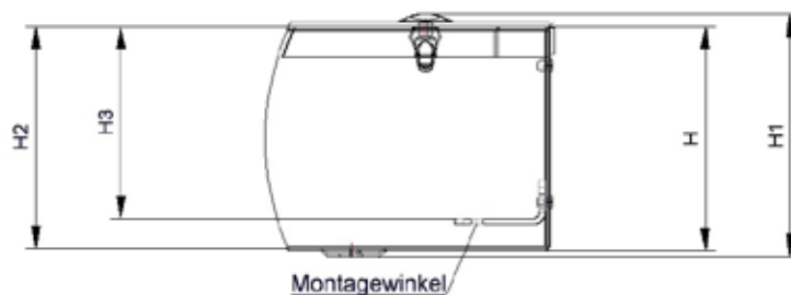
Abb. Gehäuse im Schnitt
